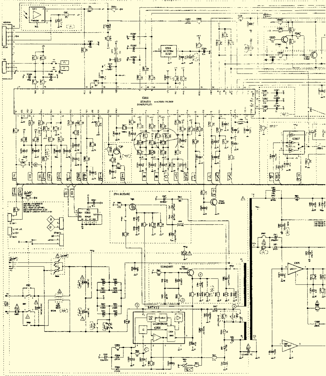
Fig. 1 - Schema elettrico della sezione SMPS comandata dall'UC3842A
